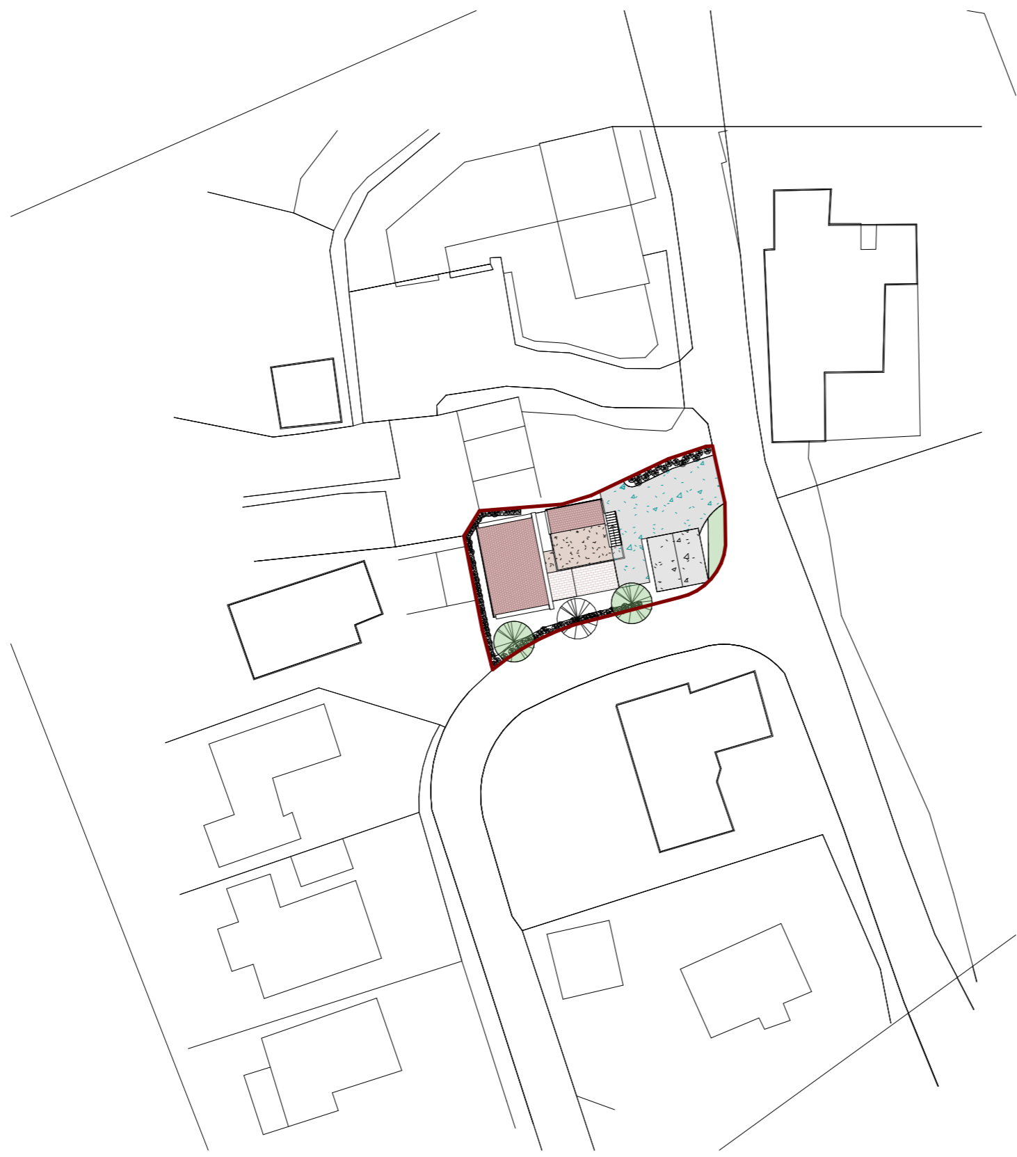
1 AREA PLAN 1 : 500
